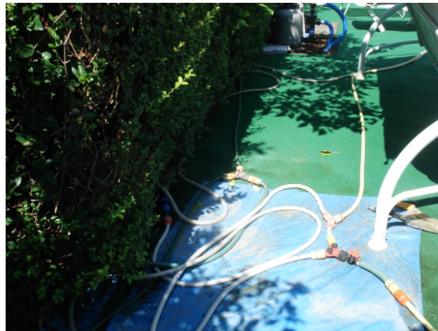
Set ventila na crevima za ručnu regulaciju protoka vode ka solaru, bazenu i tušu
